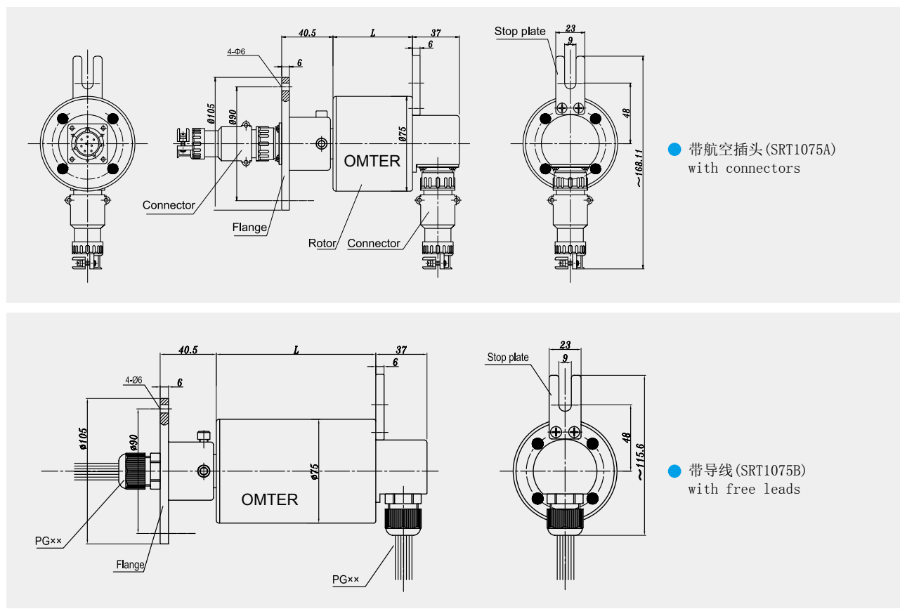
外形尺寸图 Outline Dimension
